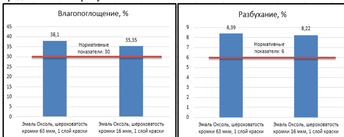
Рис. 1. Результаты исследований влияния шероховатости поверхности кромки фанеры на величину влагопоглощения и разбухания
